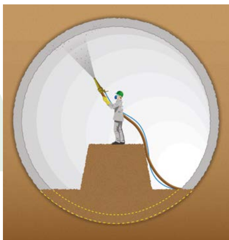
Figura 1 - Método NATM
