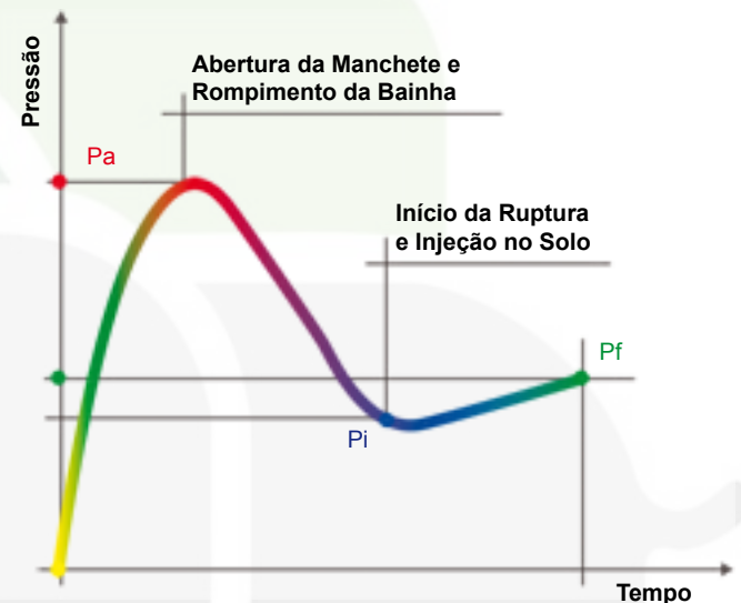
Figura 12 - Comportamento típico das pressões durante a injeção no solo
