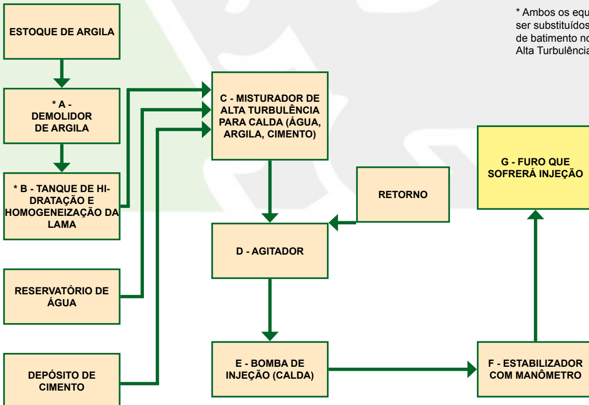
Figura 10 - Fluxograma de injeções
