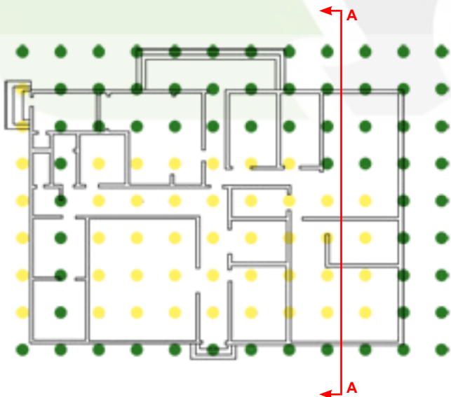
Figura 8 - Tratamento de fundação de edifício
