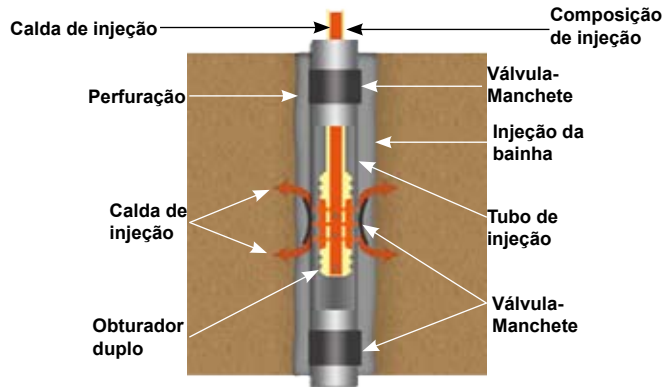
Figura 9 - Obturador duplo
