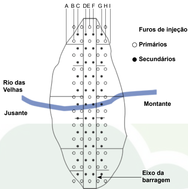
Figura 7 - Tratamento de fundação de barragem
