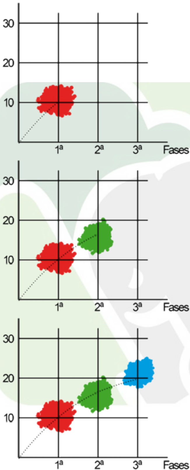
Figura 13 - Comportamento típico das pressões durante a injeção das fases
