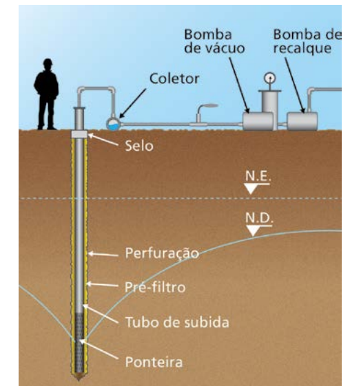
Figura 3 - Montagem geral do rebaixamento.
